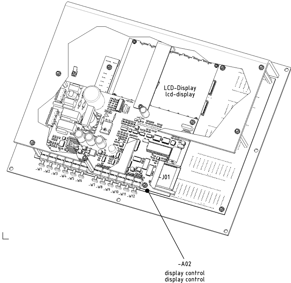
Rückansicht back view
