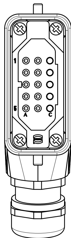
Pinbelegung / Draufsicht pin configuration / top view
