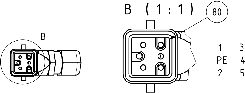
Pinbelegung / Draufsicht pin configuration / top view
