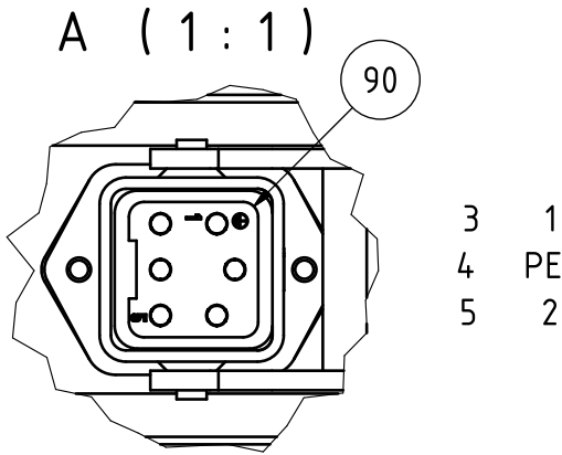
Pinbelegung / Draufsicht pin configuration / top view
